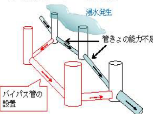
○小規模なバイパス管の設置
